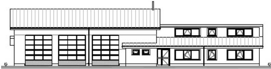
Bild Ansicht neues Feuerwehrhaus
